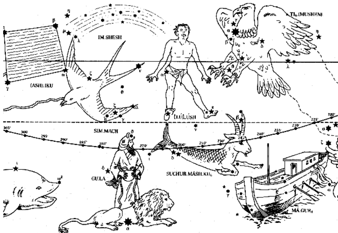
Abb 2 Die „ Wasserregion “ in den Sternen von Babylon um 2340 v.Chr. An dieser Stelle des Himmels war die Sintflut verstorbt. Aus: Papke, Werner: Die geheime Botschaft des Gilgamesch, Chaldäische Sternkarte .
