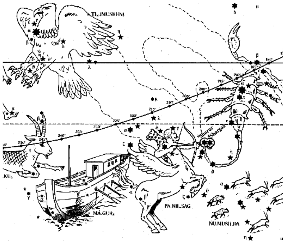
Abb. 3 Durch das „Felsentor“ am Kopf des Skorpions ( 180^\circ ) tritt Gilgamesch-Merkur in die Unterwelt ein. Vorbei am Schützen (Sagittarius), dem himmlischen Abbild des „gewaltigen Jägers“ Nimrod, gelangt Gilgamesch erst bei 227^\circ in die „Gewässer des Todes“. Aus: Pappe, Werner: Die geheime Botschaft des Gilgamesch, Chaldäische Sternkarte .
